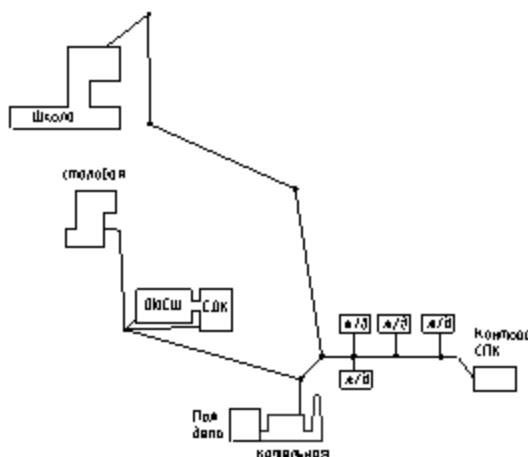
Рис. 2.3.1. Схема тепловой сети котельной села Хлопуново
